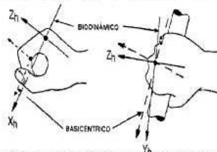
Figura 1. Sistemas bionámicos y basicéntrico de coordenadas para la mano, con indicación de los componentes de aceleración (ISO 5349 y ANSI S3-34-1986)
